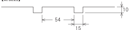
【断面図】
